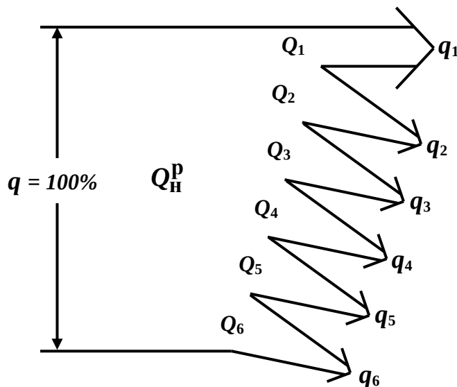
Рис. 4.2. Энергетическая диаграмма котла
